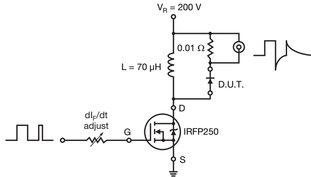
図 11 - 逆回復パラメータ試験回路
